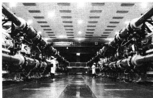
世界最大のガラスレーザー「激光Ⅷ号」
