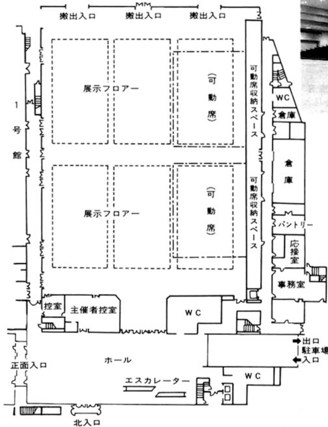
国際展示場2号館平面図 (1階)
